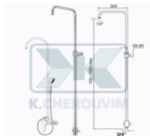
ΚΟΛΟΝΑ ΡΟΝΤΕ ΠΤΥΣΣΟΜΕΝΗ ΜΕ 1 ΣΤΗΡΙΓΜΑ ΤΟΙΧΟΥ & ΔΙΑΝΟΜΕΑ
